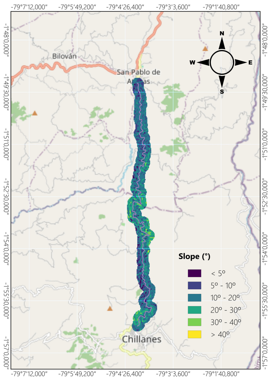
Fig. 6. Slope map.
