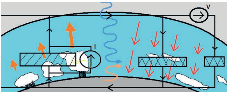
Rys. 1. Schemat globalnego atmosferycznego obwodu elektrycznego dolnej atmosfery Ziemi (jedna półkula); analogiczną część obwodu można narysować dla drugiej ziemskiej półkuli w obszarze szerokości umiarkowanych i biegunowych (poza rysunkiem). Objaśnienie: strzałkami oznaczono główne prądy obwodu – prądy Wilsona i prądy powietrze-Ziemia, a także działanie jonizujące promieniowania kosmicznego i radioaktywności; Promieniowanie kosmiczne i radioaktywność (na rysunku strzałki faliste) powodują niewielką jonizację powietrza, która wystarcza jednak do podtrzymania przepływu prądu. Napięcia elektryczne w atmosferze generują zelektryfikowane chmury konwekcyjne burzowe i opadowe, wzbudzając prądy Wilsona (pomarańczowe strzałki) płynące w górę w kierunku przewodzącej jonosfery (obszar jasnoszary). Prądy te (czerwone strzałki) wracają w obszarze pięknej pogody (prąd powietrze-Ziemia) i zamykają obwód prądów w dobrze przewodzącej powierzchni gruntu (ciemnoszary). Schemat obwodu z oporami charakteryzującymi część generatora chmurowego oraz oporności obszarów pięknej pogody, prądowym generatorem chmurowym (I) i kierunkiem przepływu prądu, jest wpisany w rysunek; gałąź obwodu w obszarze pięknej pogody obszarów polarnych zawiera zmienne (także kierunkowo) źródło napięcia (V) reprezentujące generator magnetosferyczny
