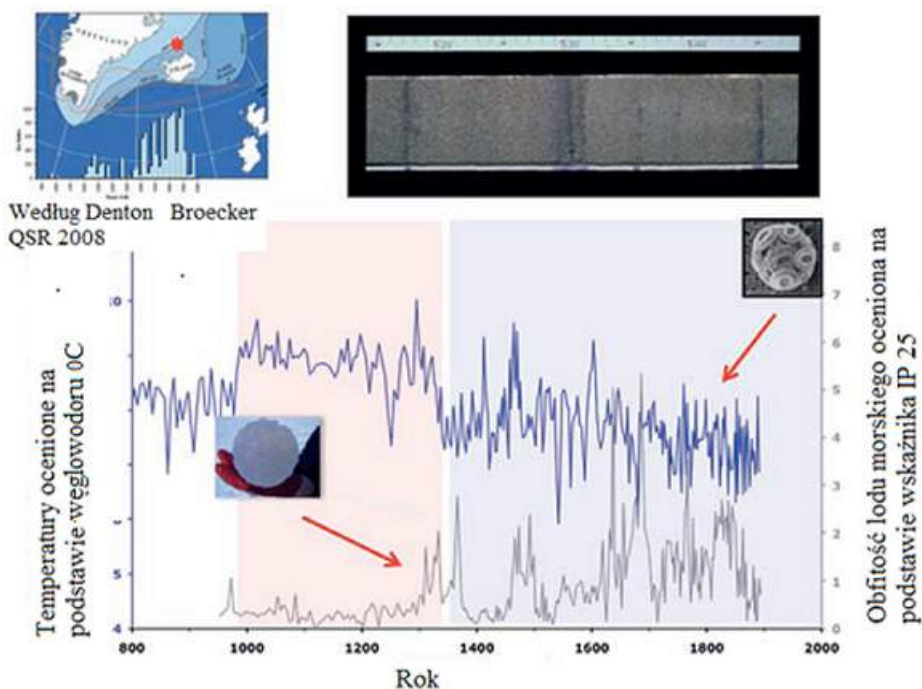
Rys. 3. Rekonstrukcja temperatury powierzchni oceanu (w ^{\circ}C ) w ciągu ostatnich 1500 lat na pełnym morzu, na północ od wybrzeży Islandii, na podstawie węglowodorów (wykres niebieski górny) i maksimum wskaźnika obfitości lodu morskiego (IP25 w ng/g, wykres szary dolny) w próbce osadów na północ od Islandii (Sicre i in., 2013). Te dane pokazują, że ochłodzenie wód podczas małej epoki lodowej (szczególnie w latach 1450-1850) było związane ze zwiększającą się trwałością lodu morskiego. Fotografia przekroju próbki osadów pozwala zidentyfikować ciemniejsze warstwy tefrytów (materiału piroklastycznego) w stosunku do reszty próbki
