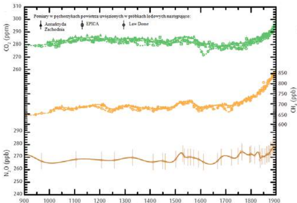
Rys. 5. Zmiany koncentracji w atmosferze: dwutlenku węgla (CO 2 ) w ppm, metanu (CH 4 ) i podtlenku azotu N 2 O w ppb, od 900 do 1900 roku, ocenione na podstawie analiz z antarktycznych próbek lodowych. Według Ciais i in. 2013
