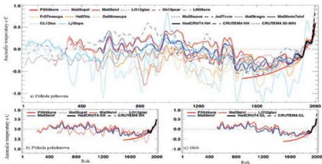
Rys. 2. Rekonstrukcja średniej rocznej temperatury: a) półkula północna, b) półkula południowa, c) glob, w ciągu ostatnich 2000 lat; kolory: czerwony – lądy na wszystkich szerokościach geograficznych, pomarańczowy – lądy poza strefą zwrotnikową, jasnoniebieski – lądy i oceany poza strefą zwrotnikową, niebieski ciemny – lądy i oceany na wszystkich szerokościach geograficznych. Temperatura zmierzona uśredniona, kolor: czarny – temperatura powierzchni lądu i oceanu (HadCRUT4); temperatura powietrza nad powierzchnią lądu i oceanu (CRU), a tylko nad lądem (CRUTEM4). Wszystkie serie przedstawiają anomalie w °C w stosunku do średniej 1881-1980 (linia pozioma wykropkowana) i wyrównane jako średnie konsekwentne 50-letnie. Według Masson- Delmotte i in. (2013)
