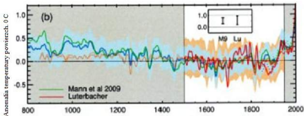
Rys. 7. Symulacje anomalii temperatury w ciągu ostatnich 1000 lat w Europie z przyjęciem danych z modelu klimatycznego uwzględniającego wymuszenia antropogeniczne i naturalne (Goosse i in., 2012). Badanie udziału wymuszeń zewnętrznych spójnych z symulacjami i z rekonstrukcjami wykonano w odniesieniu do okresu 1500-1950. Wykorzystano dwa zestawy danych z Europy: zestaw danych (kolor czerwony) odpowiada tylko danym lądowym (Luterbacher i in., 2004, „Lu” we wstawce) i dane (kolor zielony) wspólne dane lądowe i morskie (Mann i in., 2009, „M9” we wkładce). Wykres przerywany odpowiada danym instrumentalnym. Symulacje najlepiej dopasowane do rekonstrukcji Luterbachera i in. (2004), przedstawiono kolorem pomarańczowym mocnym, z zakresem przedziału niepewności w kolorze pomarańczowym jasnym są spowodowane zmiennością wewnętrzną, to znaczy nieltumaczącą się wymuszeniami uwzględnianymi w modelowaniu. Włączenie do modelowania danych Goosse i in. (2012), wymuszone rekonstrukcją Mann i in. (2009), jest przedstawione kolorem niebieskim, z przedziałem niepewności (kolor jasny niebieski). Wszystkie dane są pokazane w stosunku do średniej z okresu 1500-1950. Współczynniki skali wykorzystywane do wykrycia wymuszeń w symulacjach i w rekonstrukcjach oraz ich przedział ufności na poziomie 90% (M9 i Lu), są podane w ramce na rysunku
